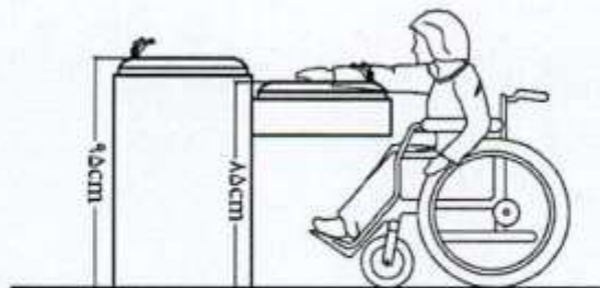
شکل شماره ۵۰: آبخوری دسترس‌پذیر در دو ارتفاع
