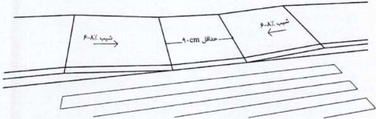
شکل شماره ۳۳: رمپ‌جدول موازی
