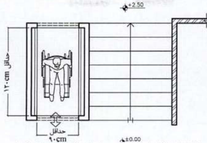
شکل شماره ۶۷: ابعاد بالابر عمودی برای طی ارتفاع ۲۰۰ تا ۲۰۰ سانتیمتر
