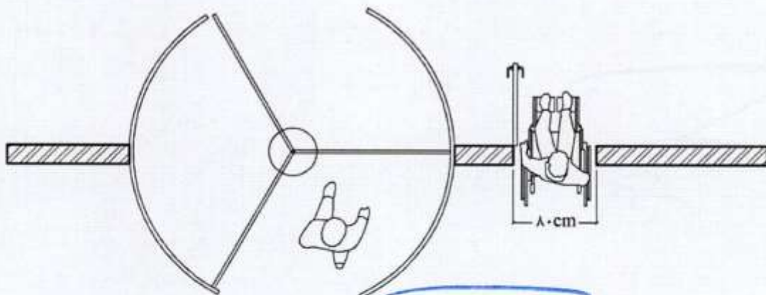
شکل شماره ۷۰: وجود یک لنگه در لولایی کنار در کردن
