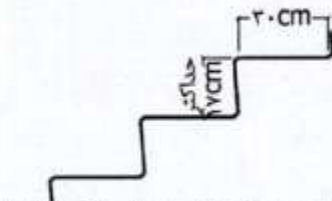
شکل شماره ۵۶: کف و ارتفاع پاخور پله‌ها
