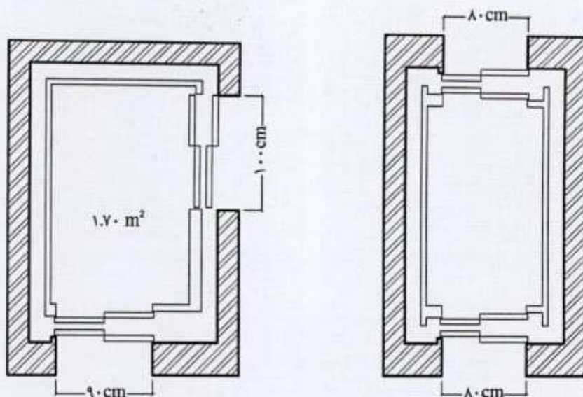
شکل شماره ۶۳: محل قرارگیری در آسانسور (الف) و (ب) آسانسورهای مختلف
