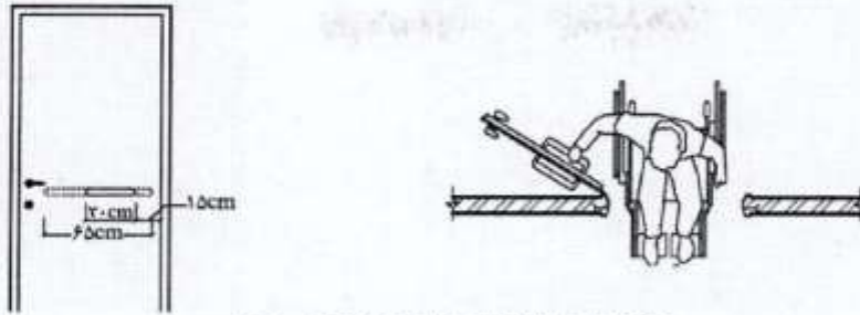
شکل شماره ۷۴: ابعاد میله دستگرد کمکی روی در
