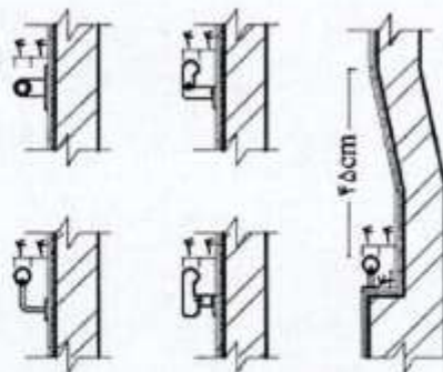
شکل شماره ۷۵: ابعاد مقطع عمودی میله دستگرد
